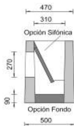
ARQUETA IMBORNAL SIN FONDO
